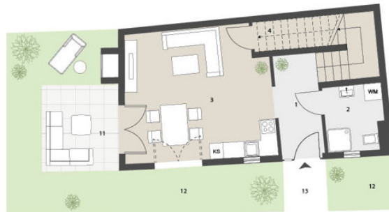
ERDGESCHOSS
