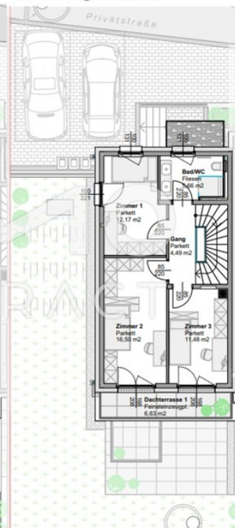
1. Obergeschoss
