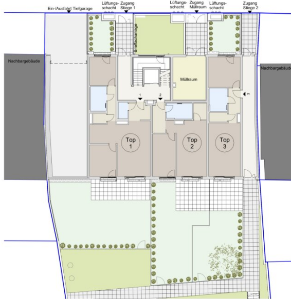
ERDGESCHOSS STRASSENBAUKÖRPER 1 : 200
