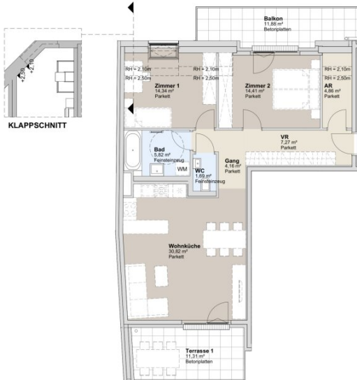
1. DACHGESCHOSS STRASSENBAUKÖRPER
