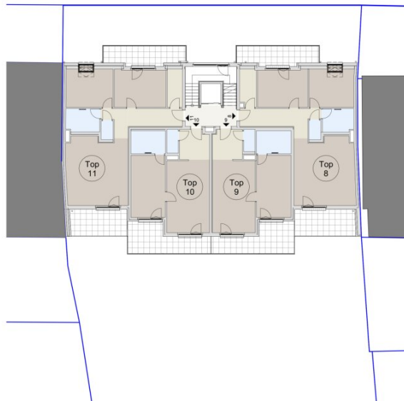
1. DACHGESCHOSS 1 : 200
