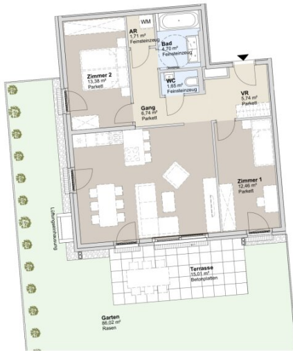
ERDGESCHOSS GARTENBAUKÖRPER
