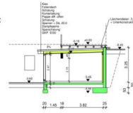
SCHNITT B - B
