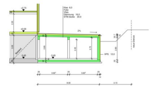
SCHNITT C - C
