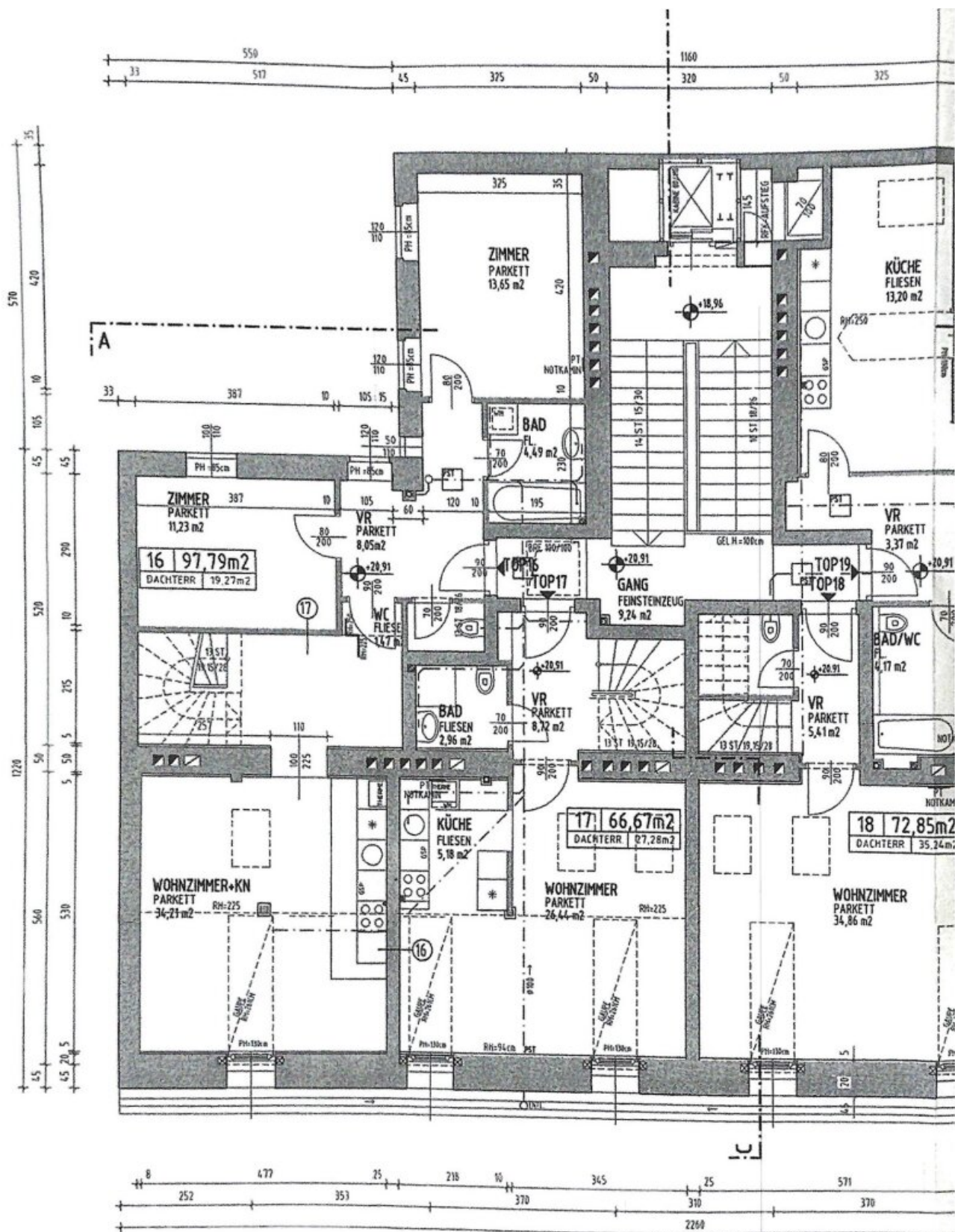
GRUNDRISS DACHGESCHOSS
