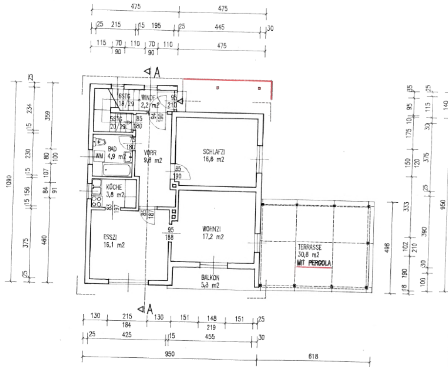
LAGEPLAN 1 : 2880
