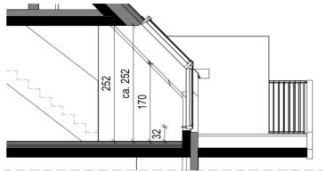
Schnitt 39.A
