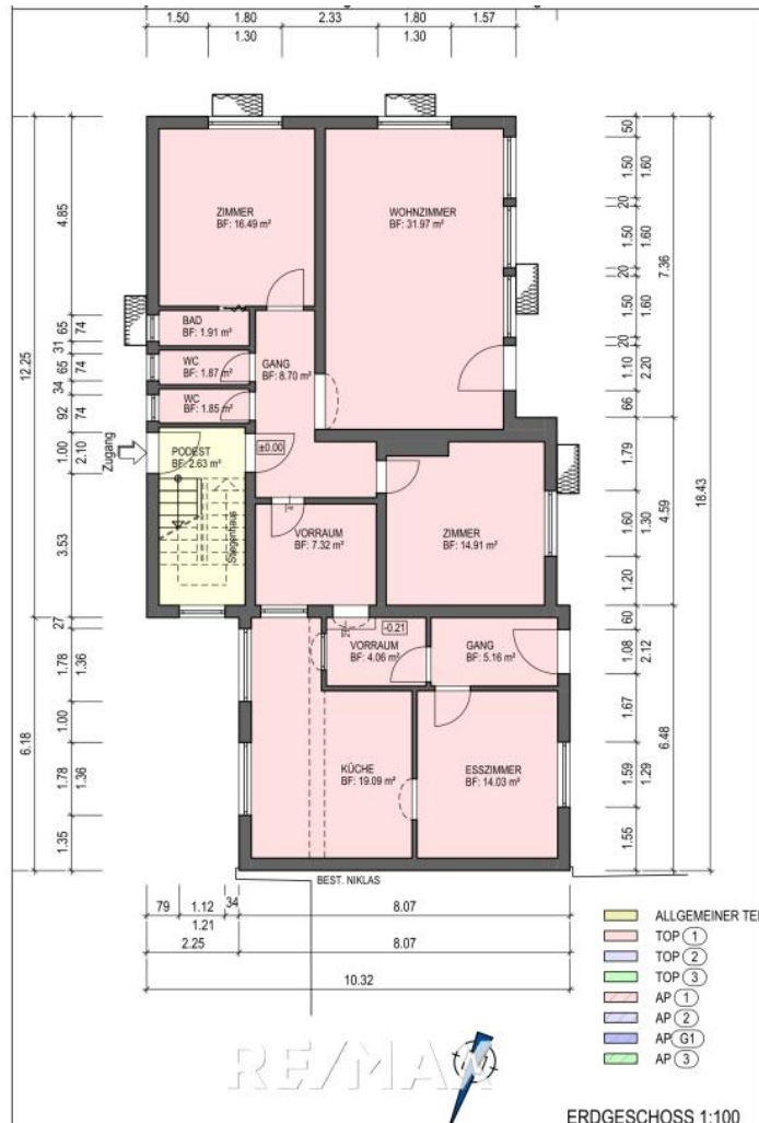
ERDGESCHOSS 1:100
