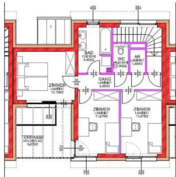
1.OBERGESCHOSS
