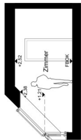
Schnitt
