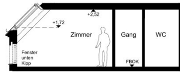
Schnitt
