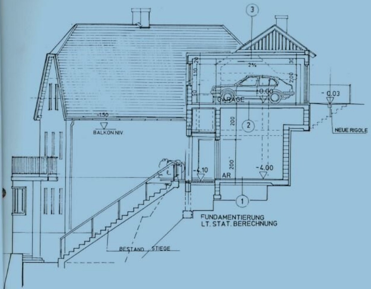
SCHNITT 3 - 3
