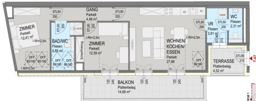
Grundriss 4 OG:
