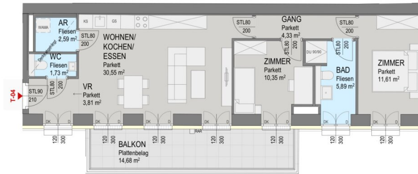
Grundriss 2 OG:
