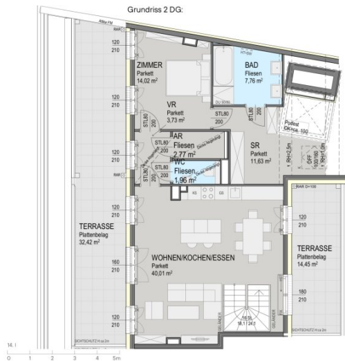
Grundriss 2 DG:
