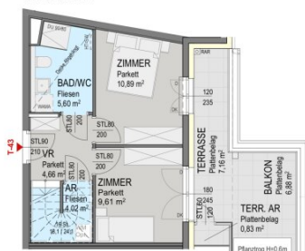
Grundriss 1 DG:
