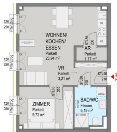
Grundriss 4 OG:
