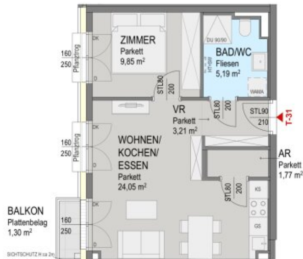
Grundriss 3 OG:
