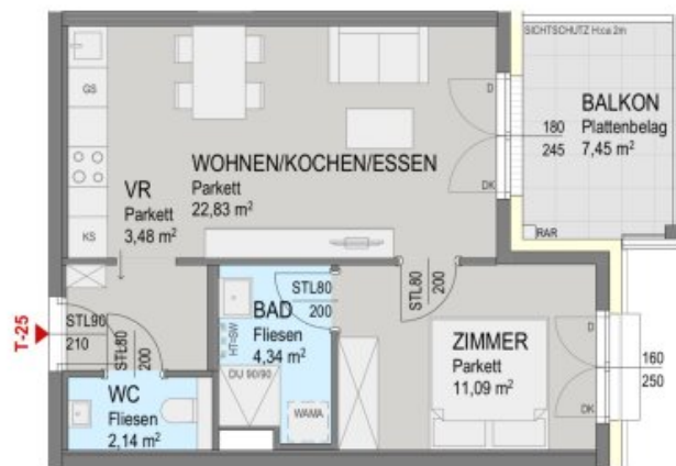
Grundriss 3 OG:
