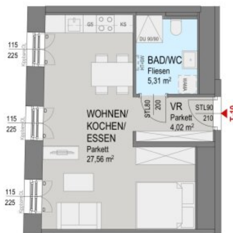
Grundriss 1 OG:
