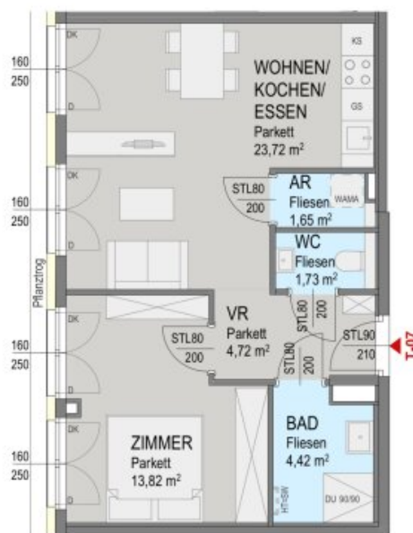
Grundriss 1 OG:
