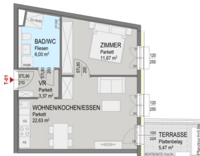
Grundriss 1 OG:
