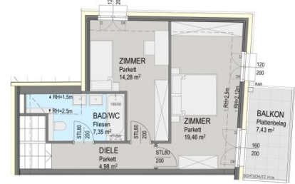
Grundriss DG:
