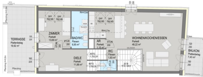
Grundriss 1 OG:
