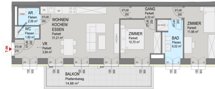
Grundriss 3 OG:
