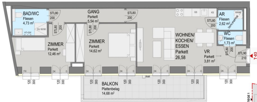
Grundriss 2 OG:
