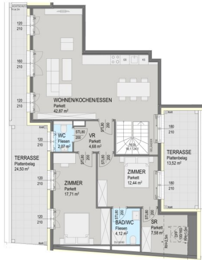
Grundriss 2 DG:
