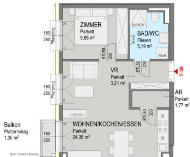
Grundriss 4 OG:
