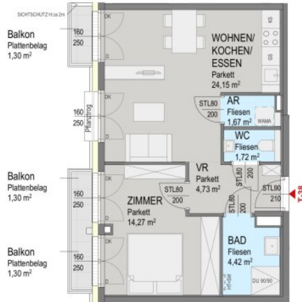
Grundriss 4 OG:
