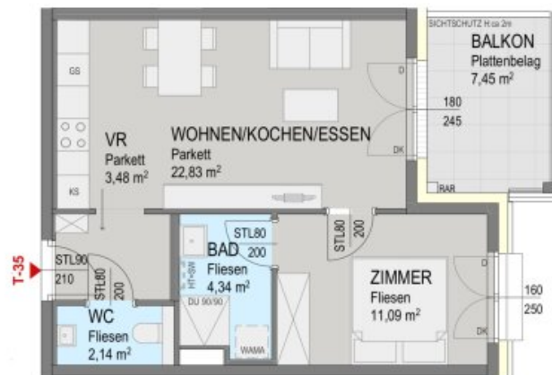
Grundriss 4 OG:
