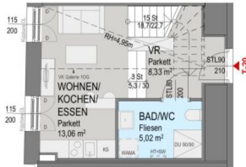
Grundriss 2 OG:
