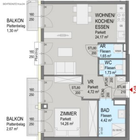
Grundriss 2 OG:
