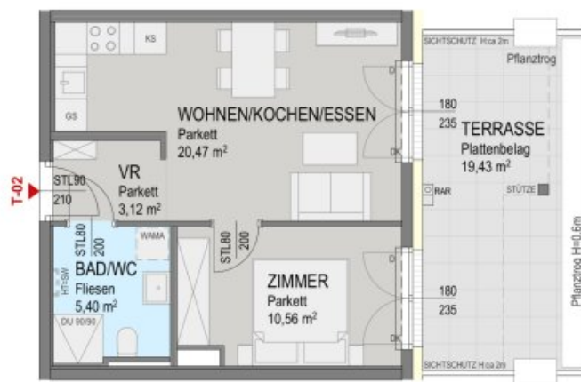
Grundriss 1 OG:
