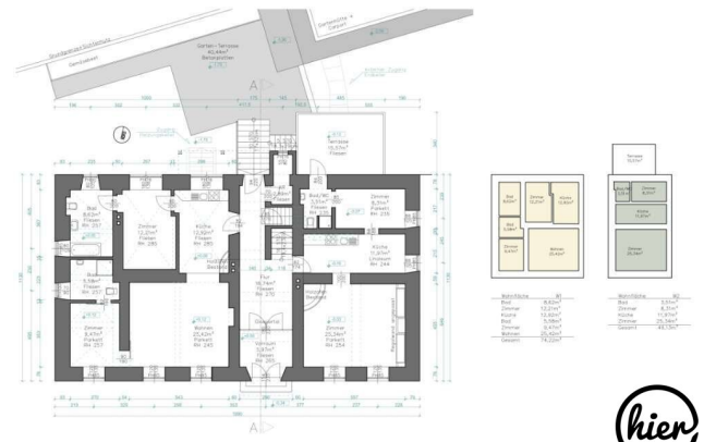
Grundriss EG, M 1:100
