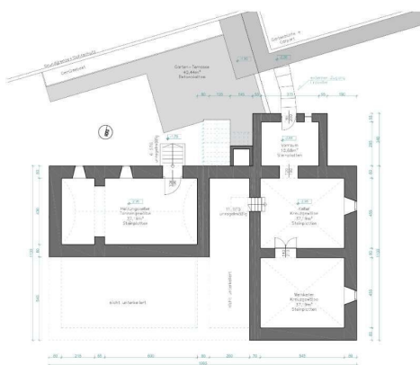
Grundriss KG, M 1:100
