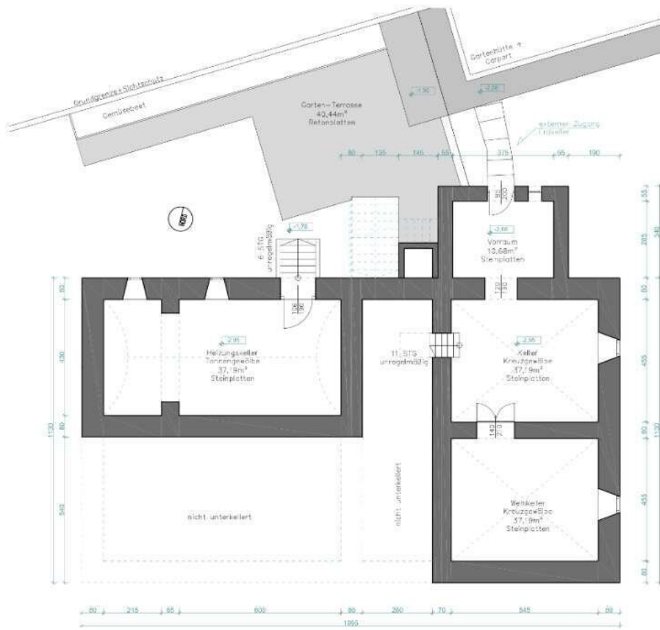
Grundriss KG, M 1:100
