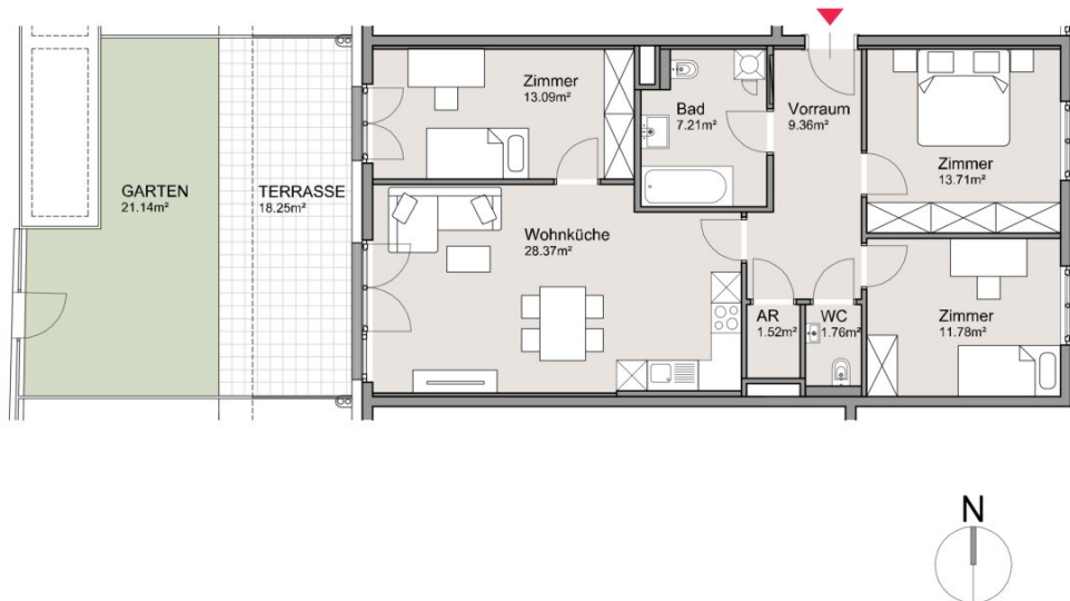
TULLNERFELD - BS5 - Wohnungsübersicht - M 1:100 - 22.12.2020
