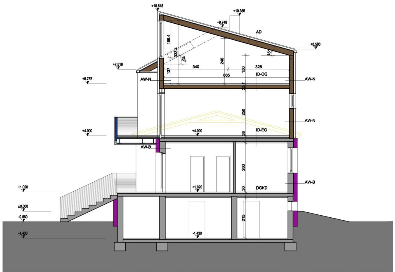
SNITT M=1:100
