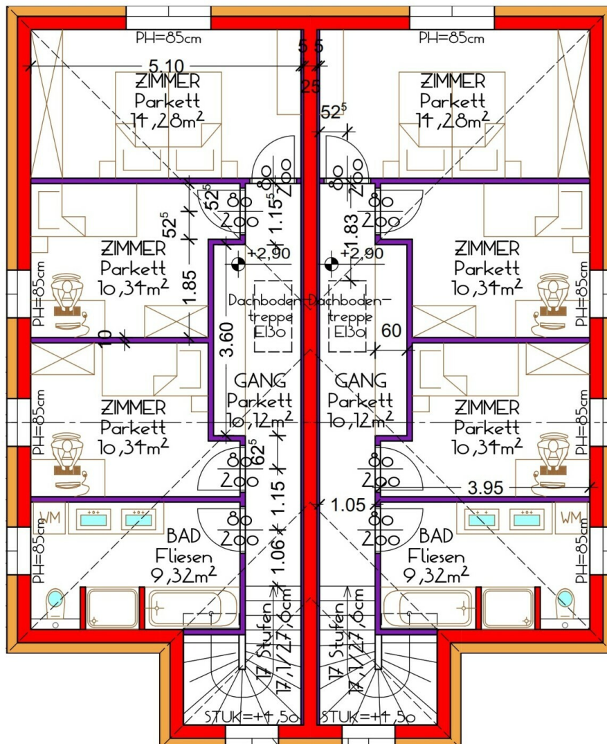
GRUNDRISS OBERGESCHOSS
