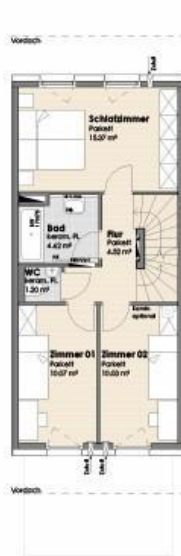
OBERGESCHOSS
