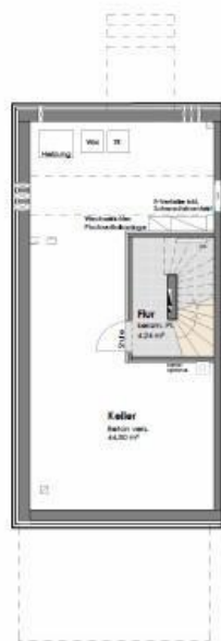
KELLERGESCHOSS
