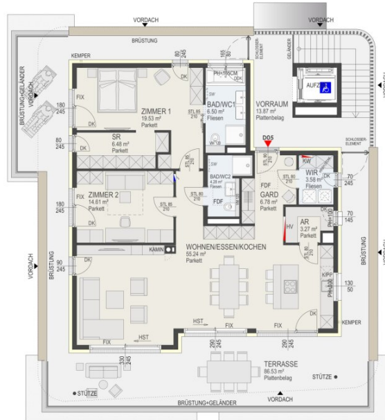
GRUNDRISSAUSSCHNITT 1.0G
