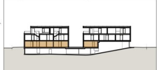
SCHNITT
