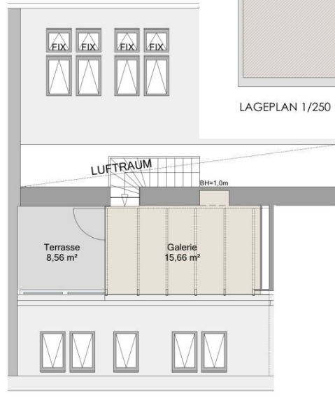
GALERIEGESCHOSS
