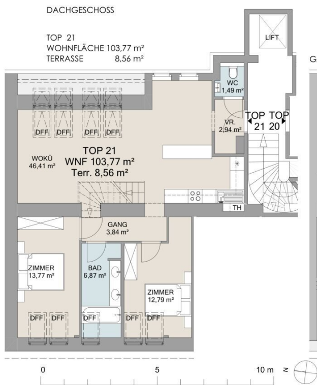
GRUNDRISS 1/100
