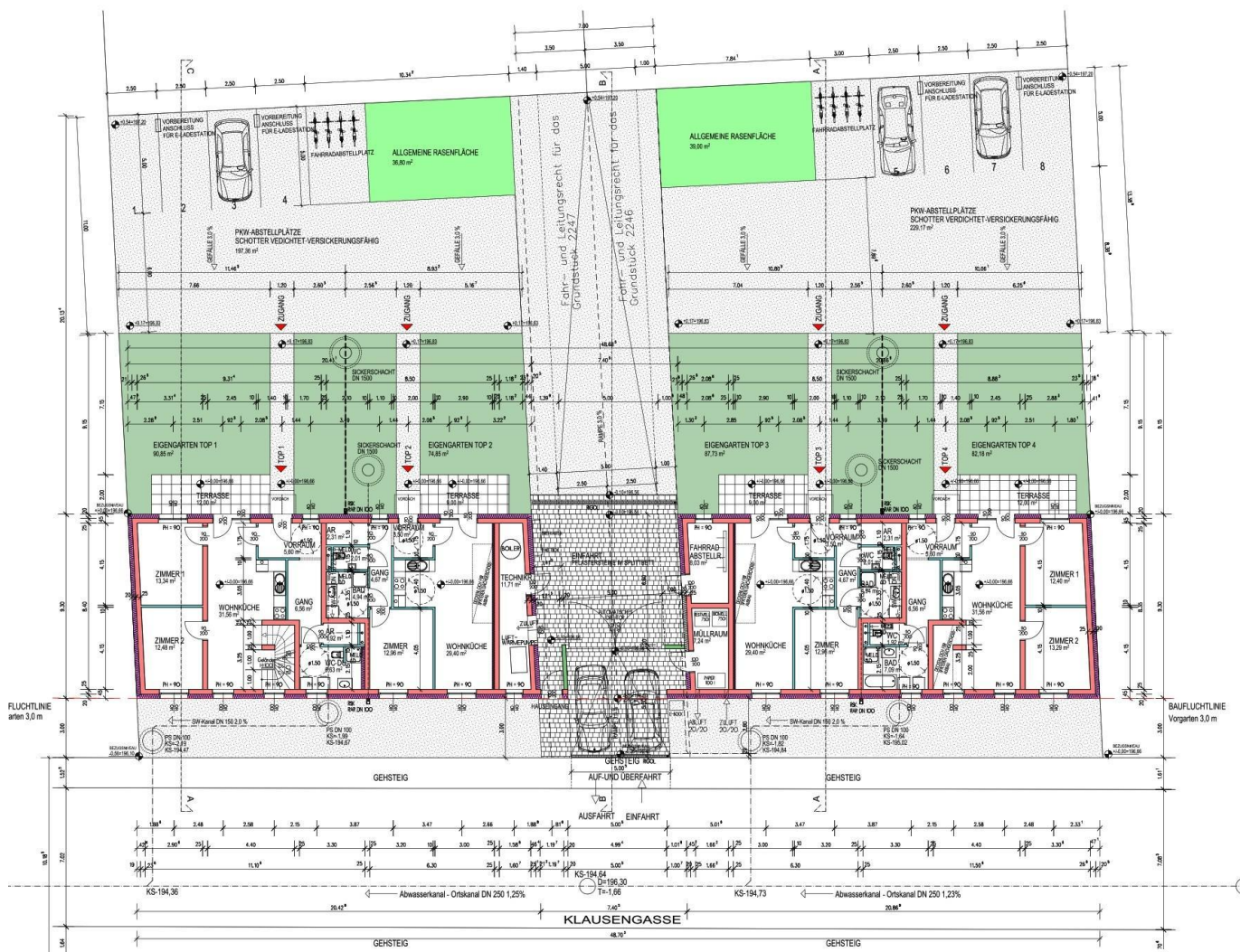
GRUNDRISS ERDGESCHOSS
