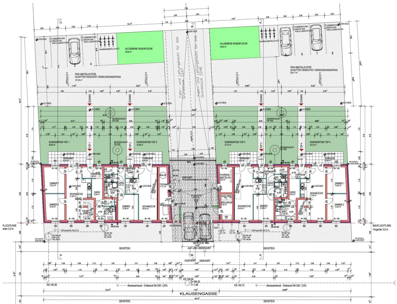
GRUNDRISS ERDGESCHOSS
