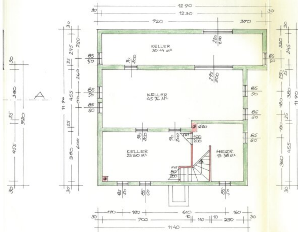
KELLER
