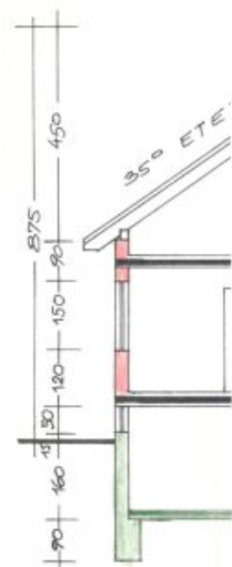
SCHNITT
