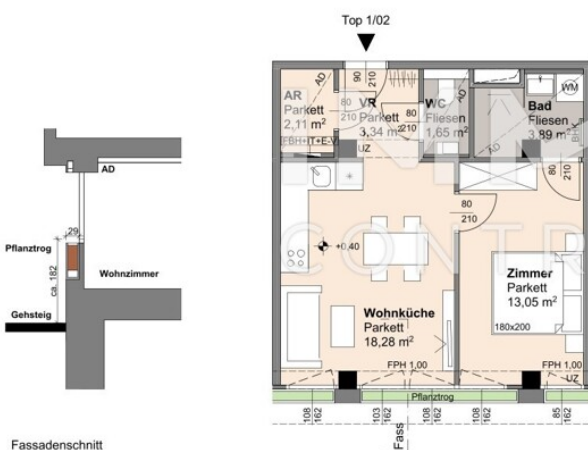
Fassadenschnitt
