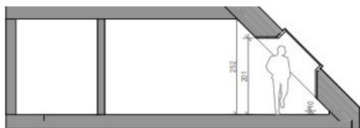
Schnitt 1-1
