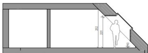
Schnitt 1-1
