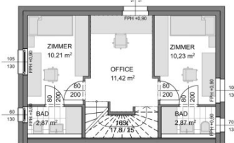
Obergeschoß
