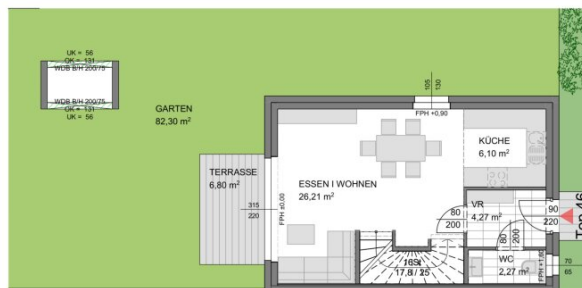
Erdgeschoß
